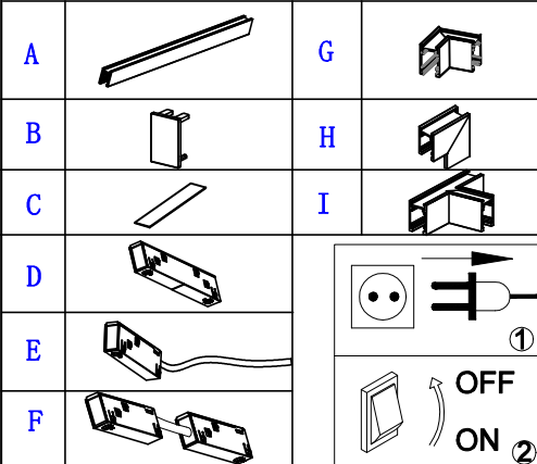
FIG-1 1013-TB-100 1013-TB-200 1013-TB-300
